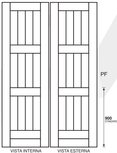
Prospetto scurone con doppio traverso centrale
