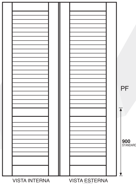
Prospetto persiana con traverso centrale
