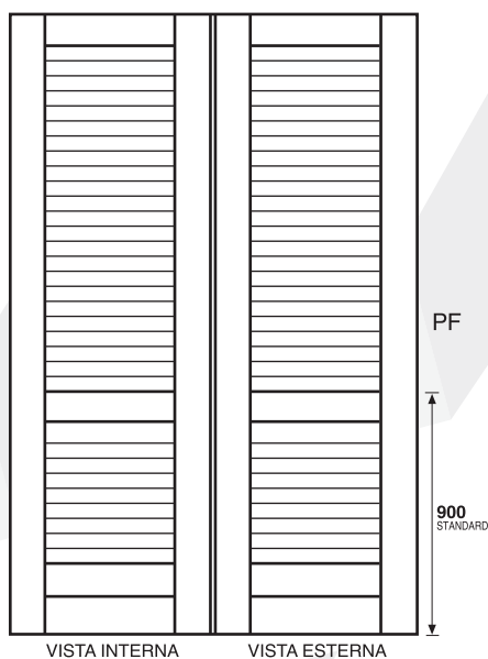
Prospetto persiana con traverso centrale
